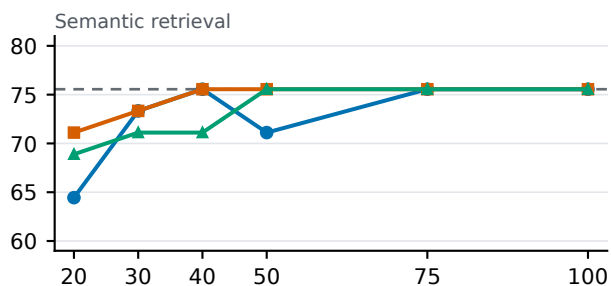
RepoQA (tiny)
