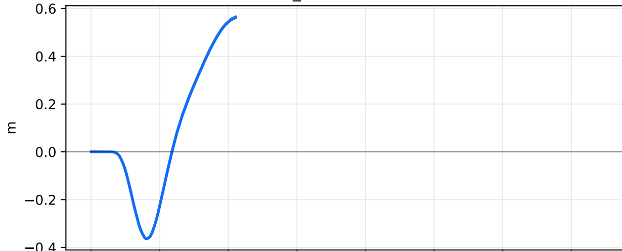
level_loiter lateral error
