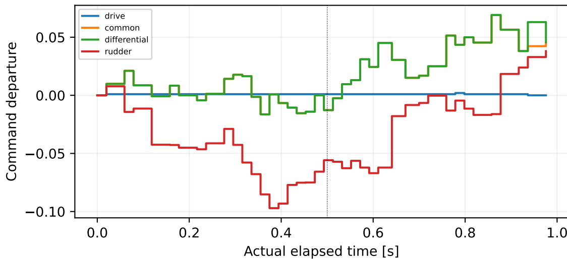
83: rudder sign=-1
