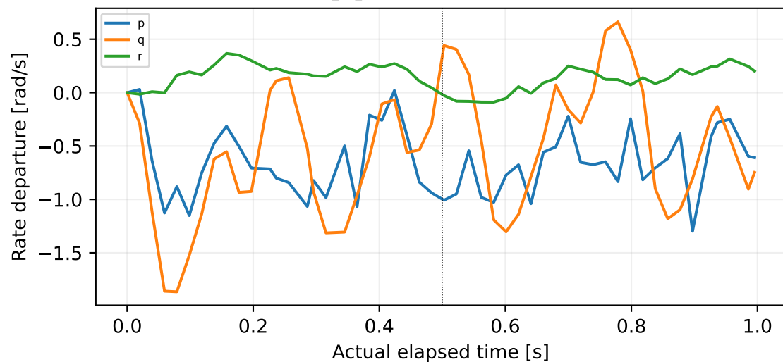
log_14_2026-9-11-18-34-58.ulg:4:1645
