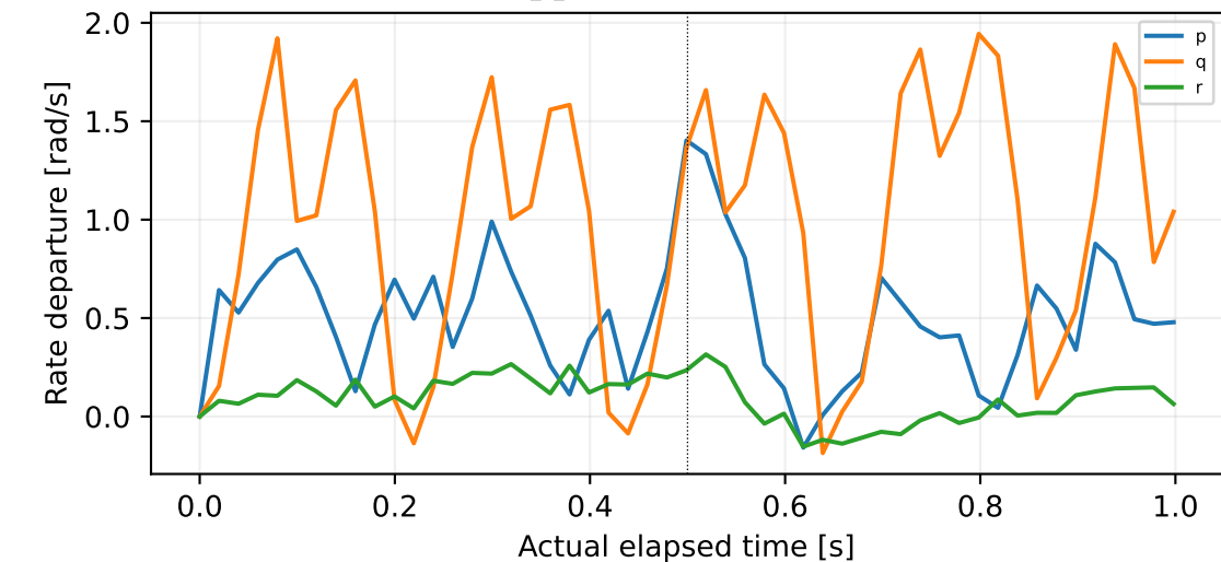
log_5_2026-9-16-18-26-48.ulg:1:415
