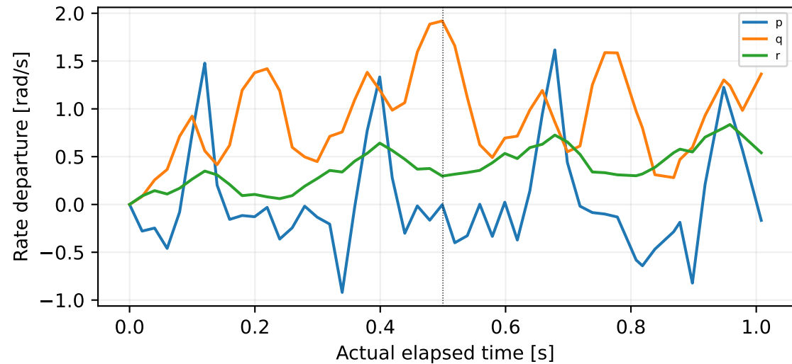
log_13_2026-9-11-18-28-08.ulg:4:25
