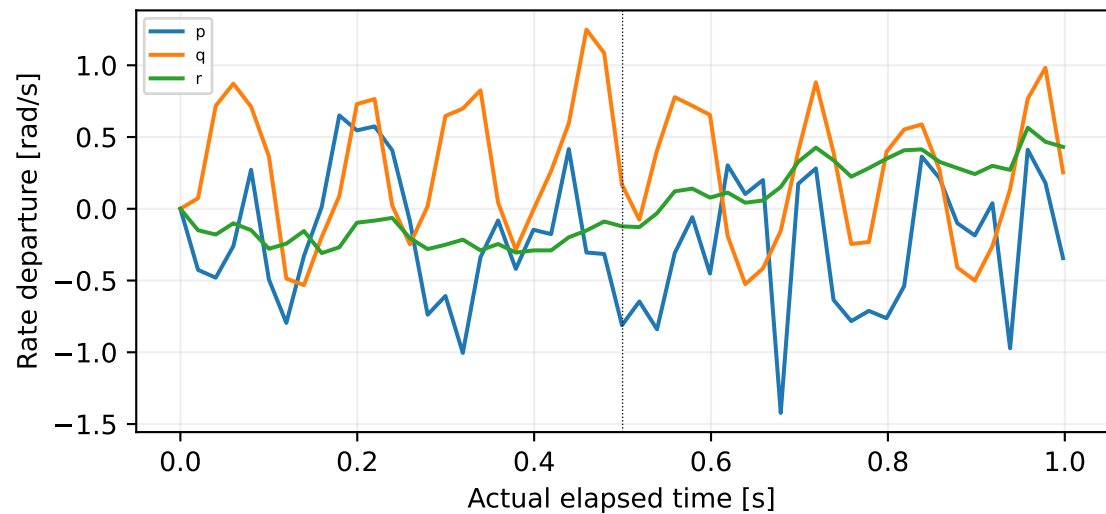
log_13_2026-9-14-18-28-32.ulg:3:895
