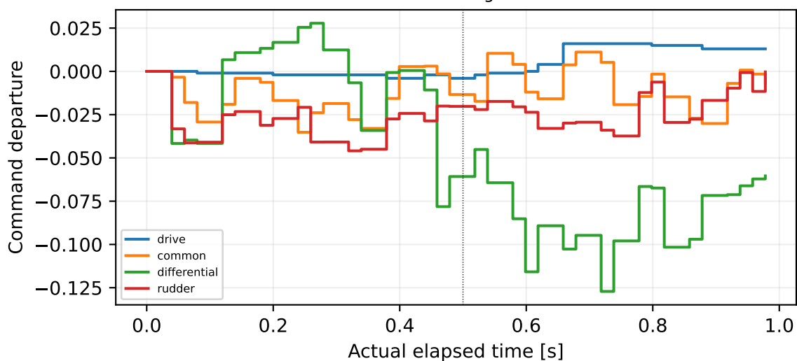
69: rudder sign=-1
