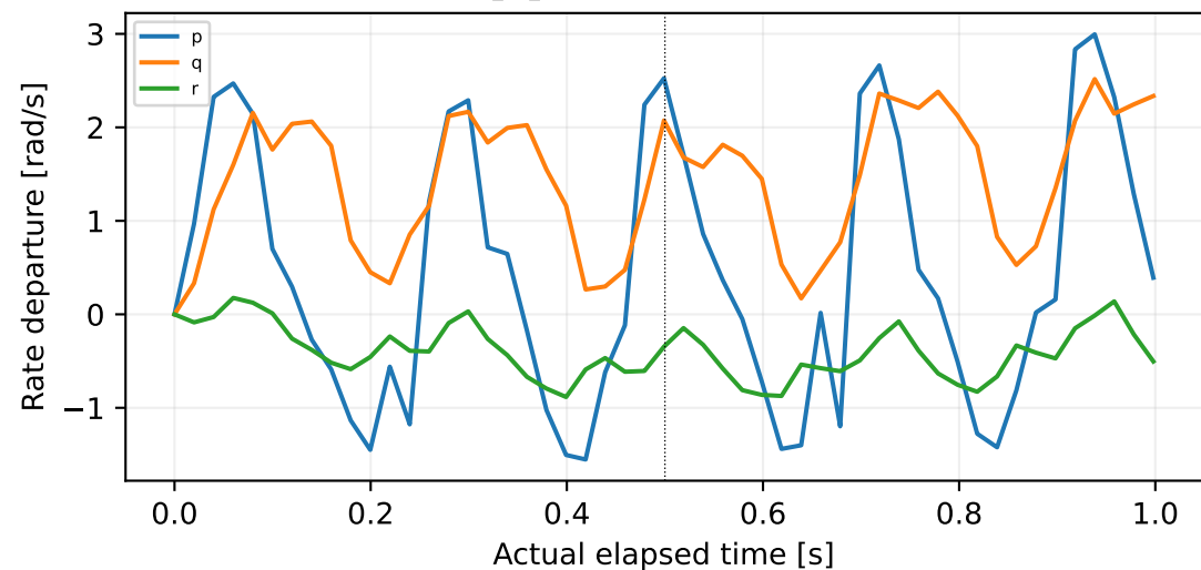
log_13_2026-9-14-18-28-32.ulg:3:715
