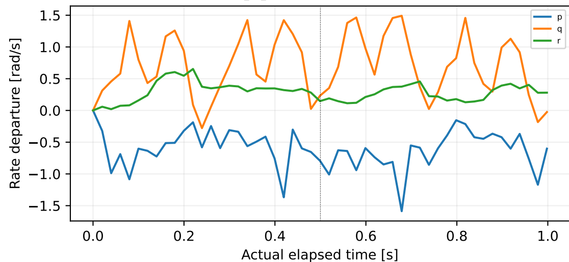
log_13_2026-9-11-18-28-08.ulg:4:885
