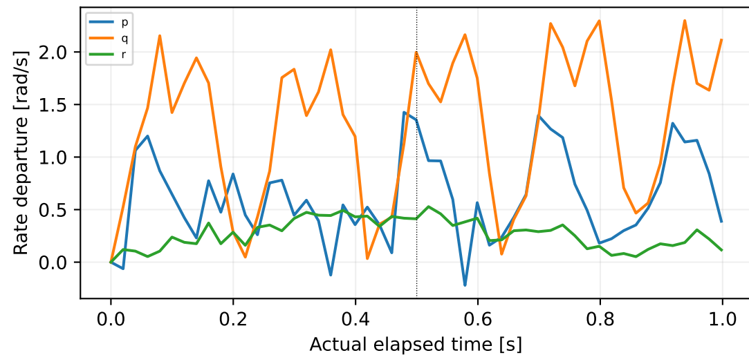
log_1_2026-9-16-18-02-34.ulg:5:45
