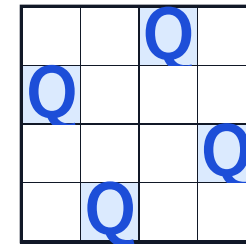
N-queens
