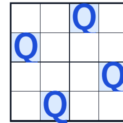
N-queens
