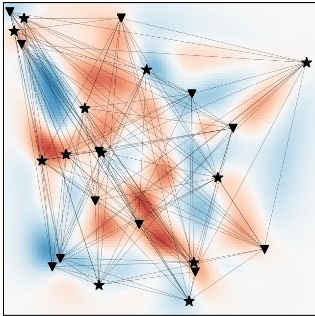
posterior expectation
