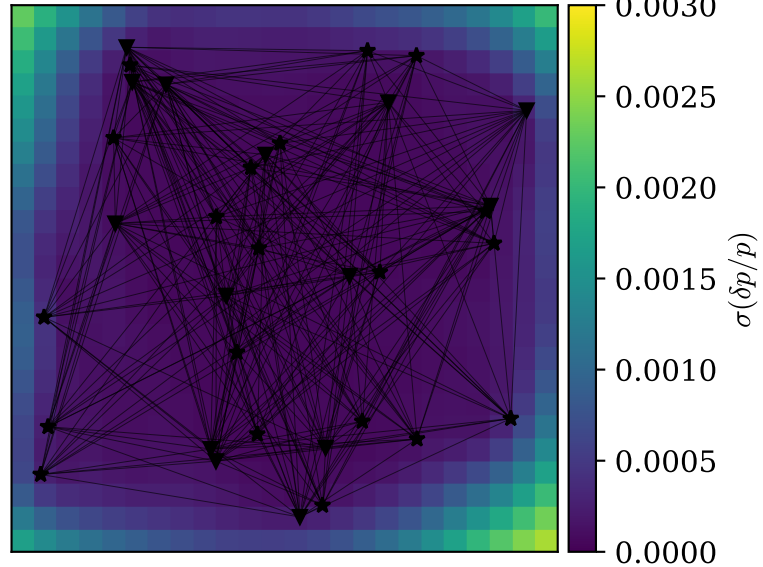
posterior standard deviation
