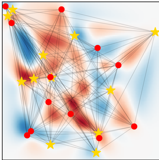
posterior expectation
