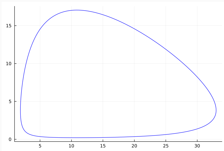
Figure 1: График численности хищников от численности жертв
