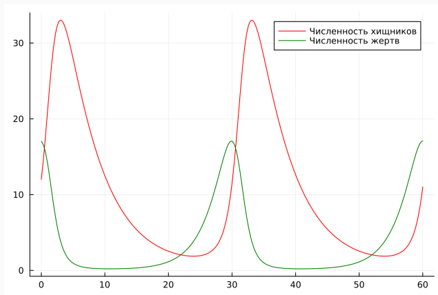
Figure 2: График численности жертв и хищников от времени
