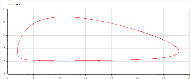
Figure 4: График численности хищников от численности жертв
