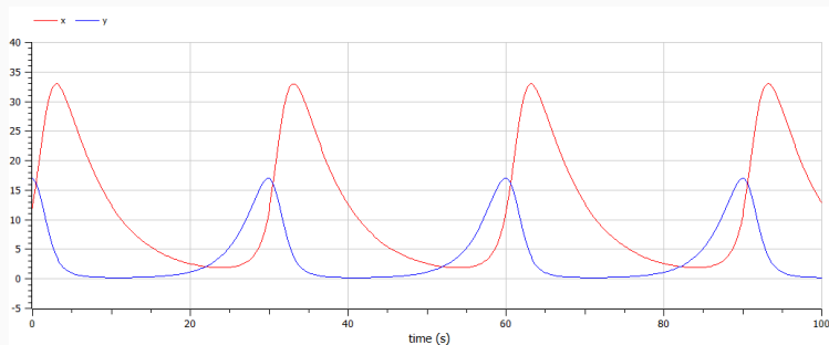
Figure 5: График численности жертв и хищников от времени
