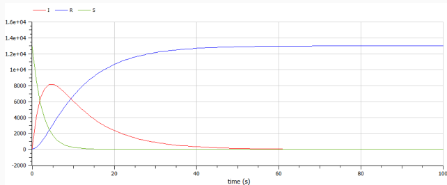
Figure 4: Графики численности особей трех групп S, I, R, построенные на Julia, для случая, когда больные могут заражать особей группы S
