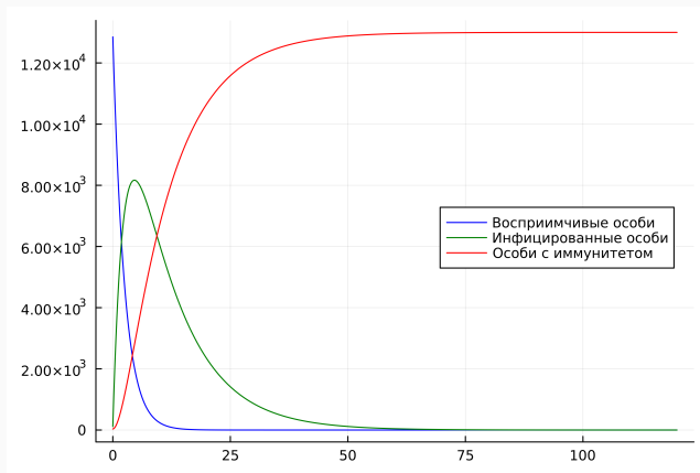
Figure 2: Графики численности особей трех групп S, I, R, построенные на Julia, для случая, когда больные могут заражать особей группы S
