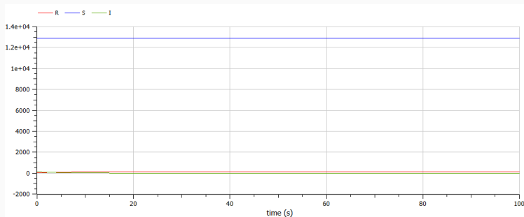
Figure 3: Графики численности особей трех групп S, I, R, построенные на Julia, для случая, когда больные изолированы
