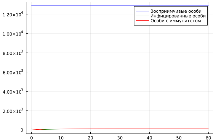
Figure 1: Графики численности особей трех групп S, I, R, построенные на Julia, для случая, когда больные изолированы
