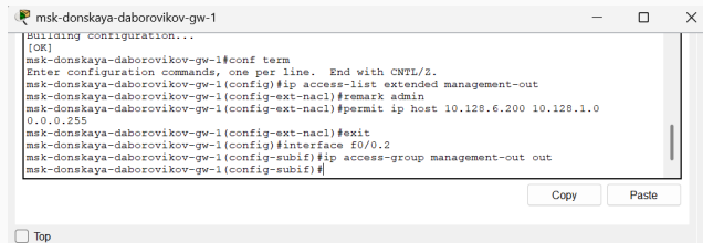
Figure 16: Настройка доступа администратора к сети сетевого оборудования ( 10.128.6.200 разрешён доступ к сети сетевого оборудования (10.128.1.0); к интерфейсу f0/0.2 подключён список прав доступа management-out и применено к исходящему трафику)
