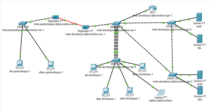
Figure 1: Подсоединение ноутбука к порту 24 коммутатора sw-4
