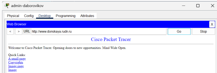
Figure 13: Проверка доступности web-сервера (через браузер) по имени
