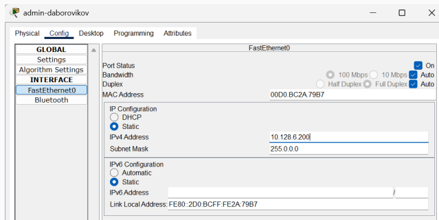
Figure 2: Присвоение оконечному устройству статического адреса 10.128.6.200, gateway-адреса 10.128.6.1 и адреса DNS-сервера 10.128.0.5
