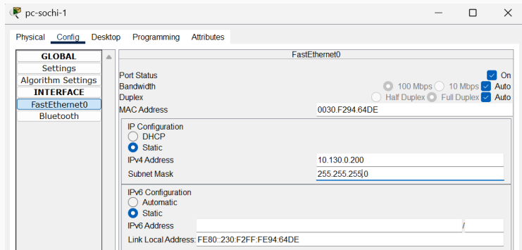
Figure 19: Присвоение адресов оконечному устройству pc-sochi-1.
