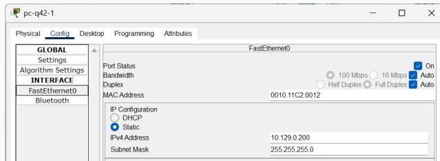
Figure 10: Присвоение адресов оконечному устройству pc-q42-1.
