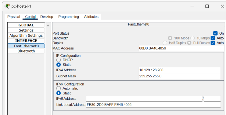
Figure 15: Присвоение адресов оконечному устройству pc-hostel-1.
