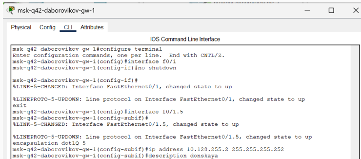
Figure 3: Настройка интерфейсов маршрутизатора msk-q42-daborovikov-gw-1.
