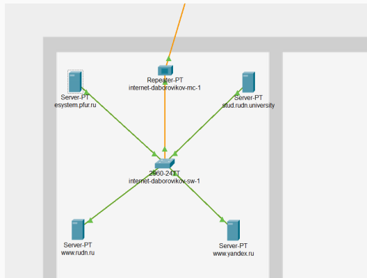
Figure 5: Оборудование в здании сети модельного Интернета
