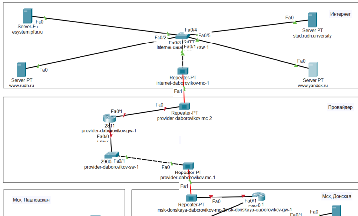
Figure 1: Схема сети с выходом в Интернет
