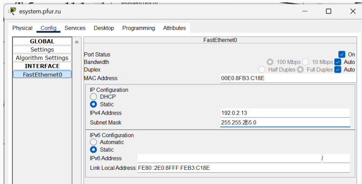
Figure 7: Прописываем IP-адреса серверам
