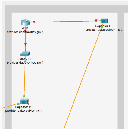
Figure 4: Оборудование в здании сети провайдера
