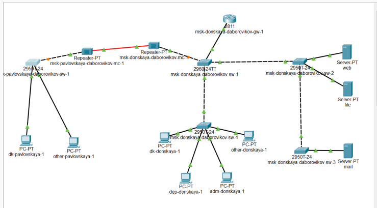
Figure 13: Подключение, оптоволокно, витая пара
