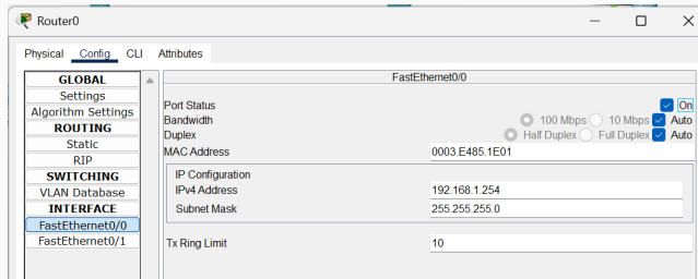
Figure 14: Настройка маршрутизатора
