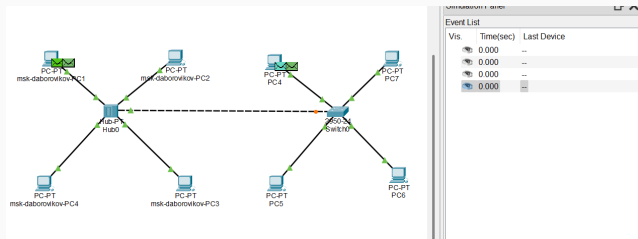
Figure 12: Сценарий с концентратором и коммутатором
