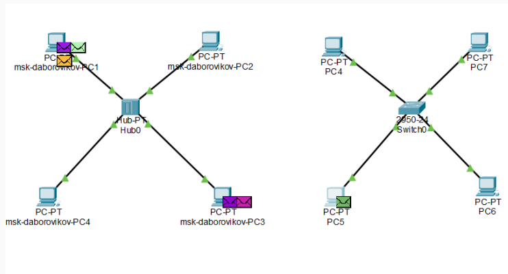
Figure 9: Схема сети с коммутатором
