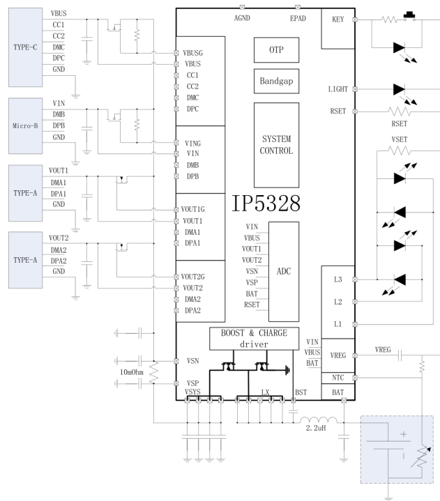
图 1 简化应用原理图(4 LED 指示电量)
