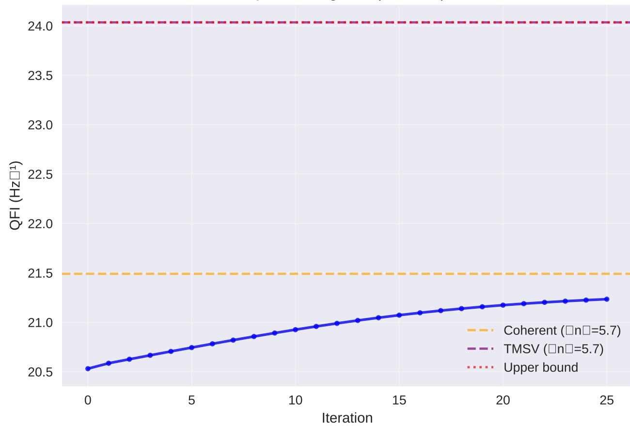
QFI Change per Step
