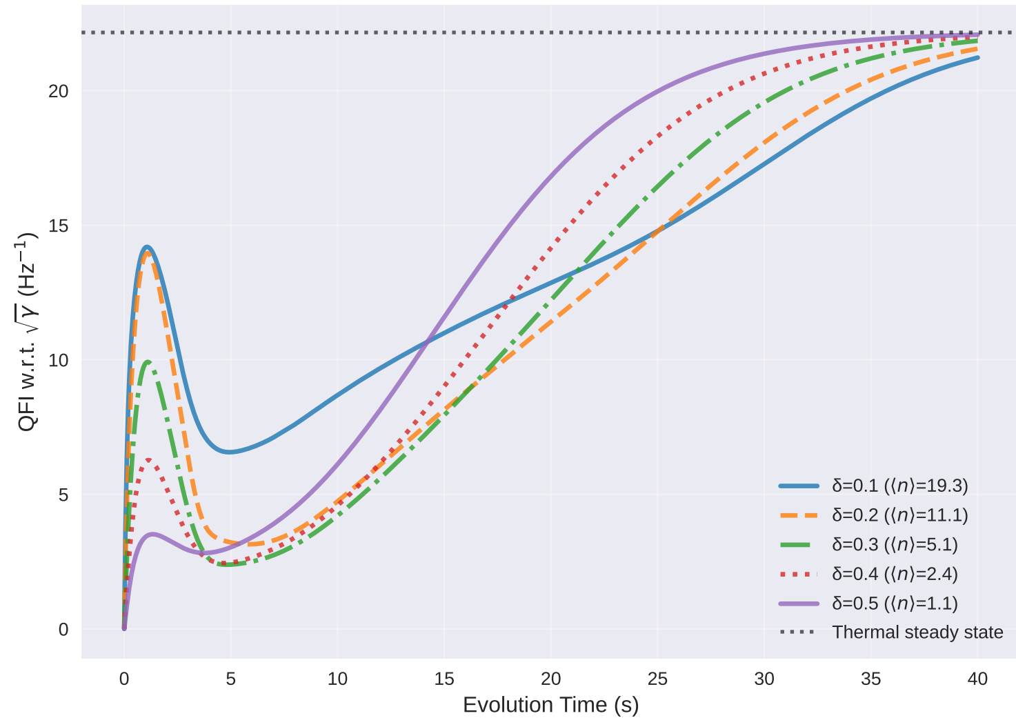
GKP State QFI: Different \delta Parameters
