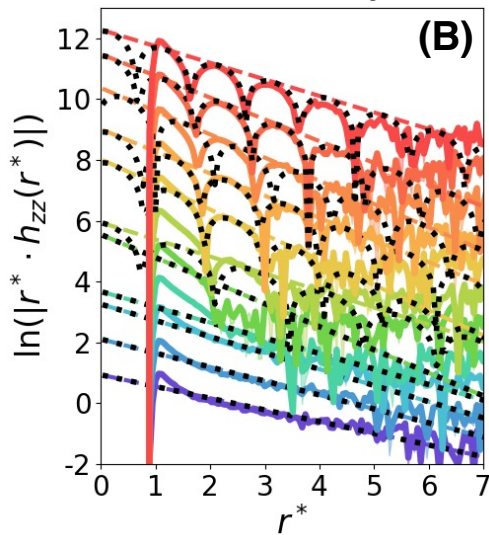
WCA electrolytes
