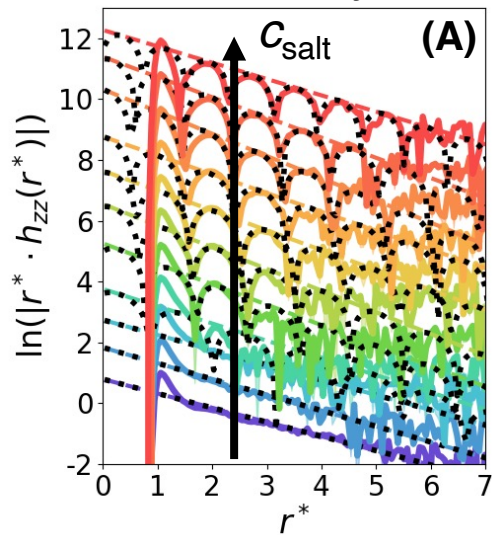
LJ electrolytes
