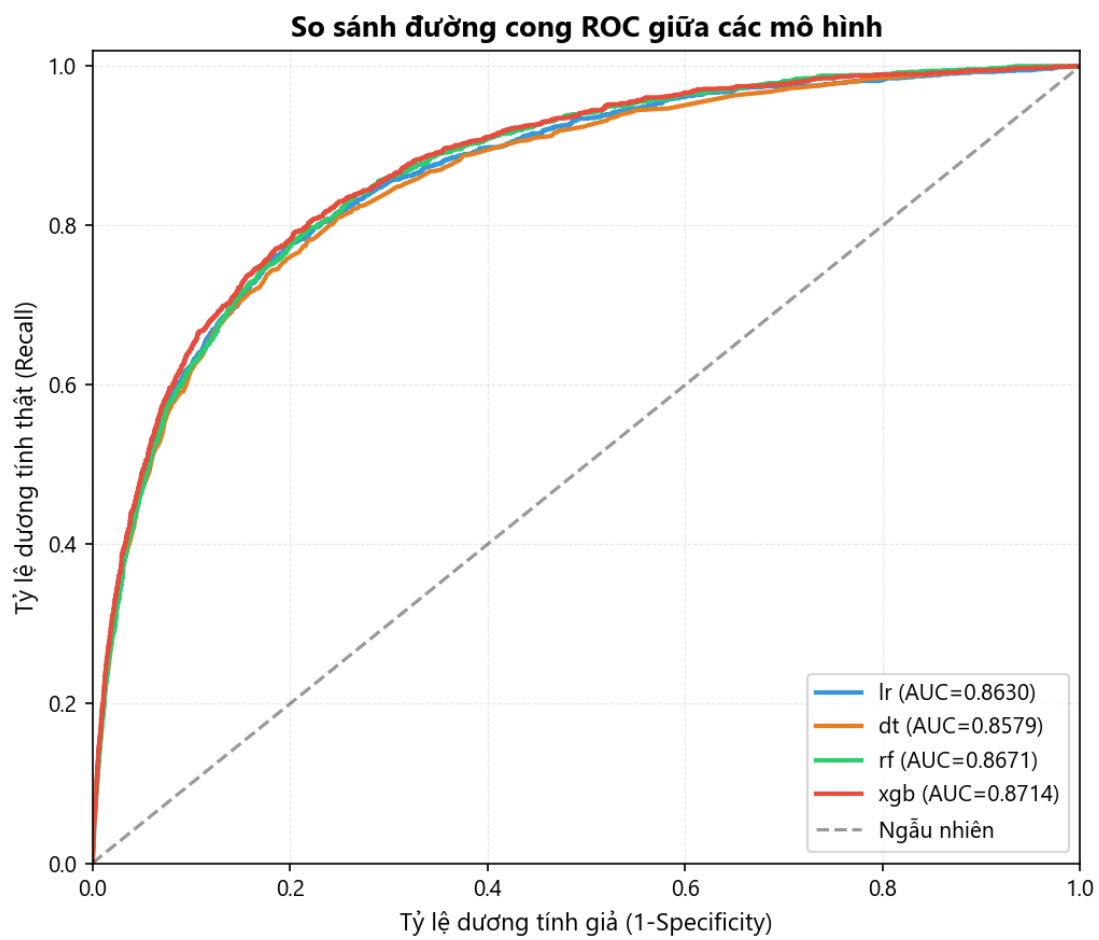
Hình 4.1: Đường ROC của bốn mô hình trên tập kiểm tra.
