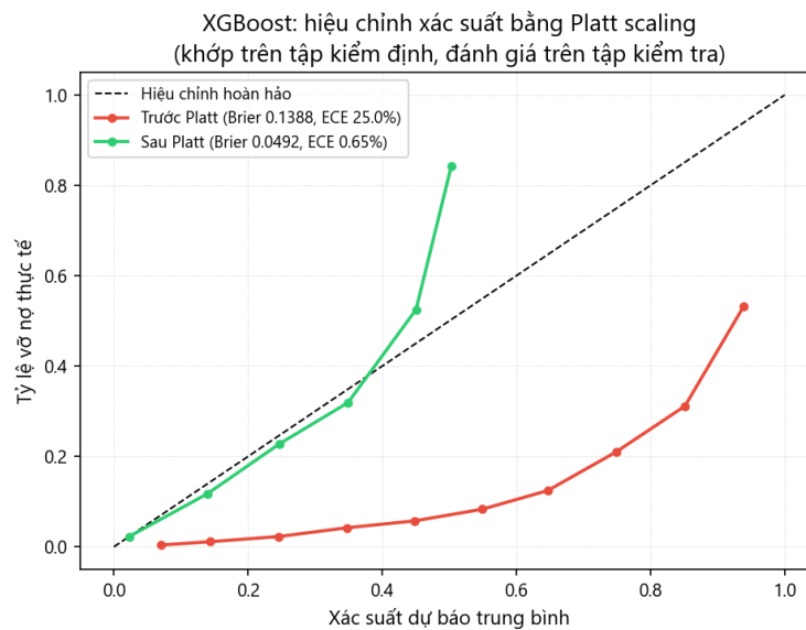
Hình 4.6: XGBoost trước/sau hiệu chỉnh Platt scaling trên tập kiểm tra.
