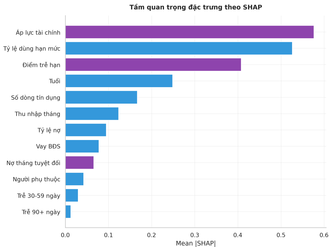
Hình 4.2: Tầm quan trọng đặc trưng theo giá trị SHAP.
