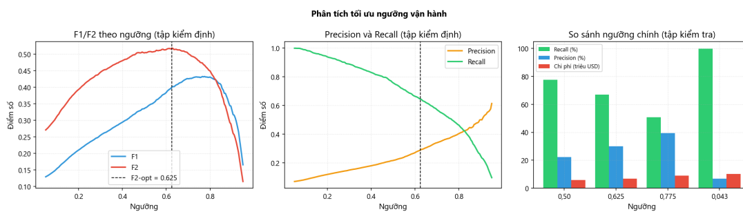
Hình 4.3: Tối ưu ngưỡng vận hành theo F_2 .
