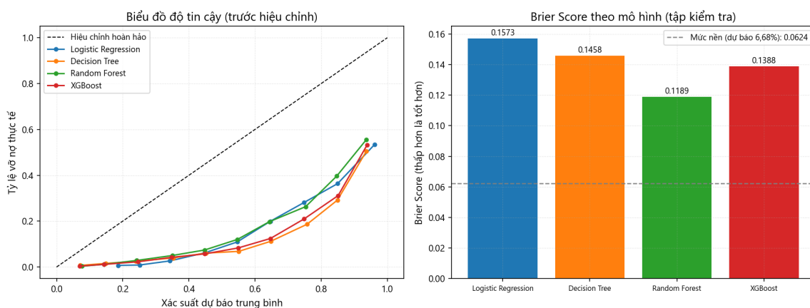
Hình 4.5: Biểu đồ độ tin cậy và điểm Brier của bốn mô hình (trước hiệu chỉnh).
