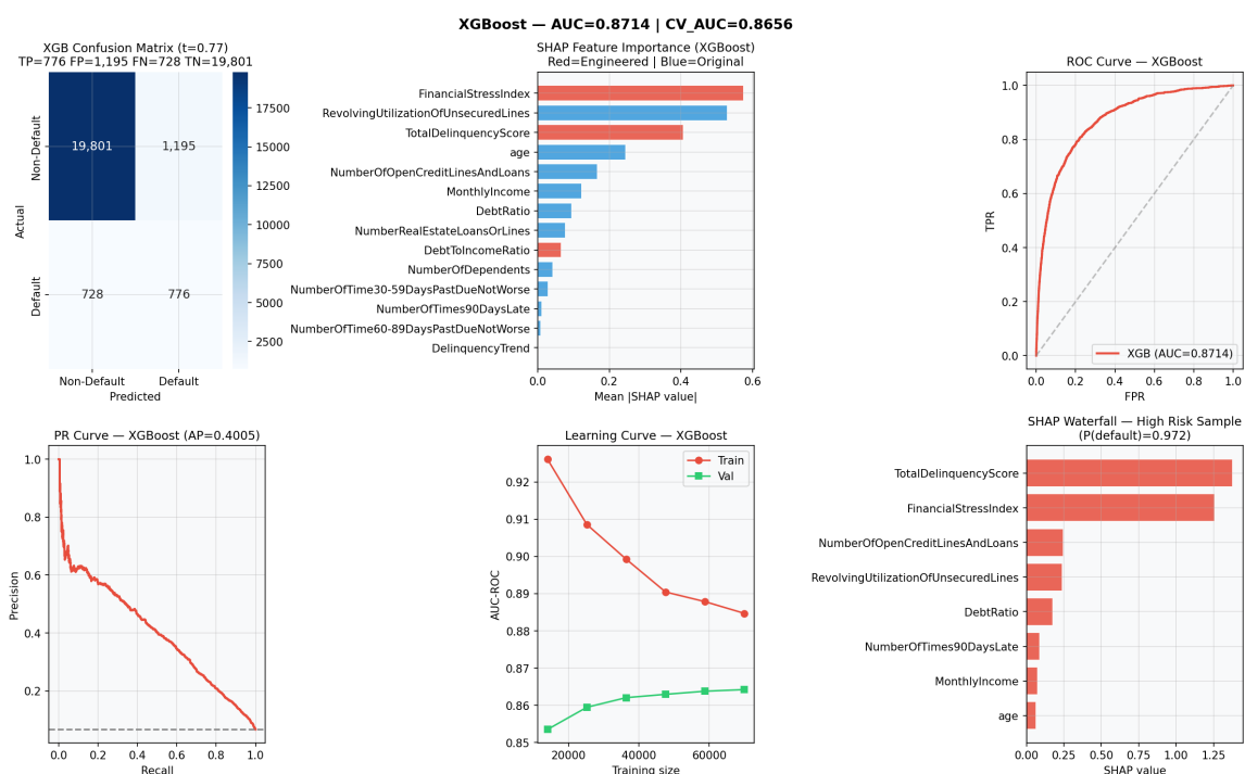
Figure 4.1. XGBoost đạt AUC = 0,8714 — đường ROC nằm xa đường ngẫu nhiên, đường PR thể hiện hiệu quả ở ngưỡng độ chính xác cao, đường cong học hội tụ sau ~ 45.000 mẫu với khoảng cách huấn luyện/xác thực = 0,021.
