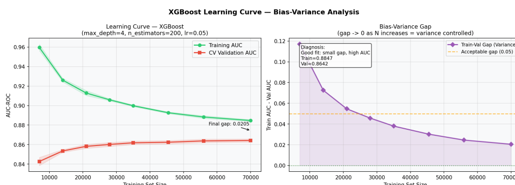
Figure 4.6. Khoảng cách train-val thu hẹp từ 0,117 (10% dữ liệu) xuống 0,021 (100% dữ liệu) — mô hình không xảy ra hiện tượng quá khớp và đã hội tụ; AUC xác thực bình ổn sau N \approx 45.000 cho thấy nút thắt cổ chai là chất lượng đặc trưng, không phải thiếu dữ liệu.
