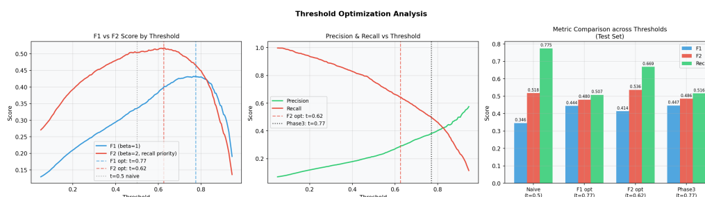
Figure 4.5. Ngưỡng F_2 -tối ưu t = 0,625 (đường đứt) đạt cân bằng tốt hơn cho bài toán tín dụng so với ngưỡng F_1 t = 0,775 — tăng Recall từ 51,6% lên 66,9%, giảm ước tính chi phí $2 M trên tập test 22.500 khách hàng.
