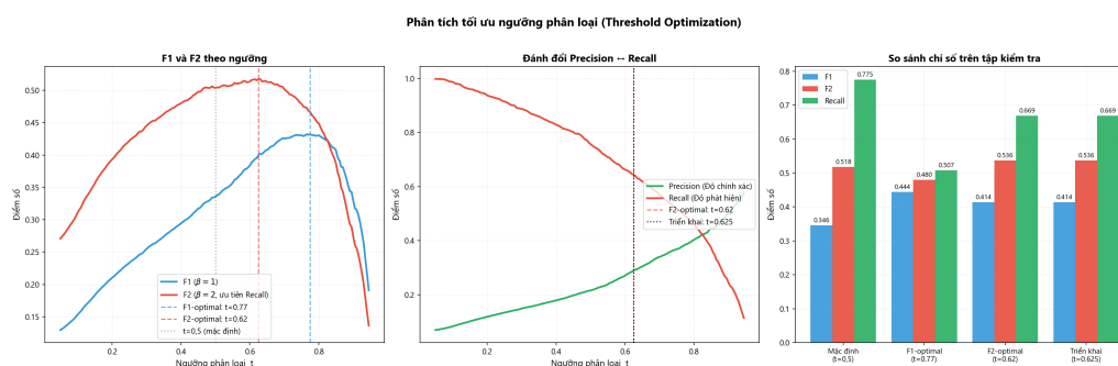
Figure 4.5. Ngưỡng F_2 -tối ưu t = 0,625 (đường đứt) đạt cân bằng tốt hơn cho bài toán tín dụng so với ngưỡng F_1 t = 0,775 — tăng Recall từ 51,6% lên 66,9%, giảm ước tính chi phí $2 M trên tập test 22.500 khách hàng.
