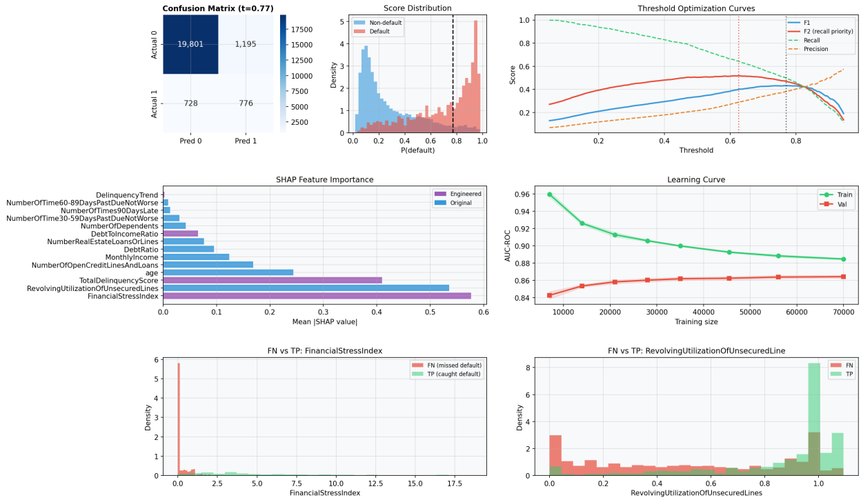
Figure 17: Bảng điều khiển phân tích tổng hợp
