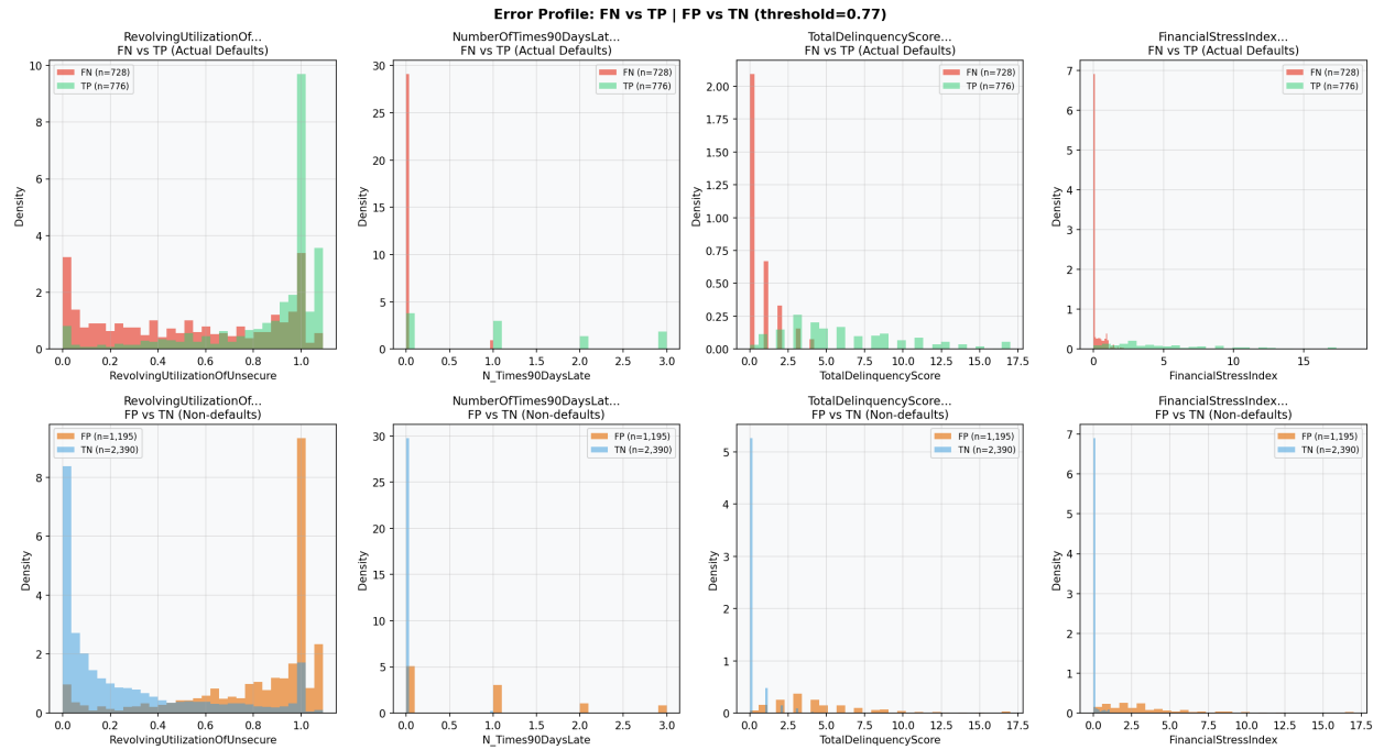
Figure 14: Hồ sơ sai số theo phân phối
