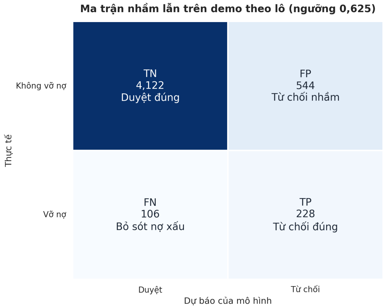
Figure 8: Ma trận nhầm lẫn trên demo theo lô
