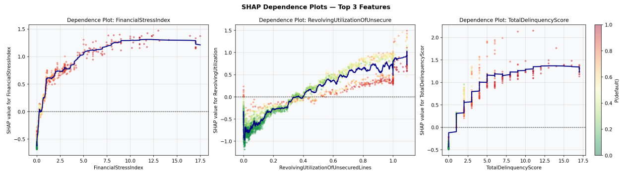
Figure 12: SHAP dependence cho đặc trưng chính
