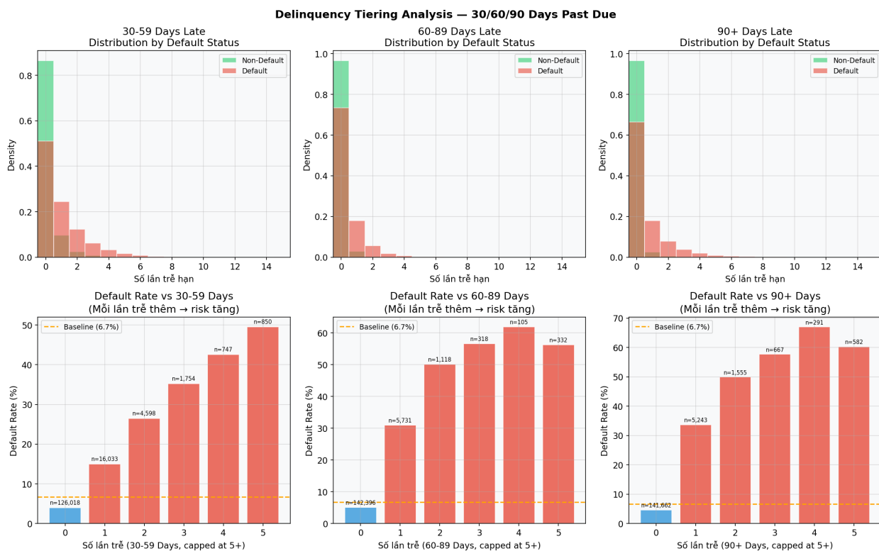
Figure 3: Phân tích nhóm trễ hạn
