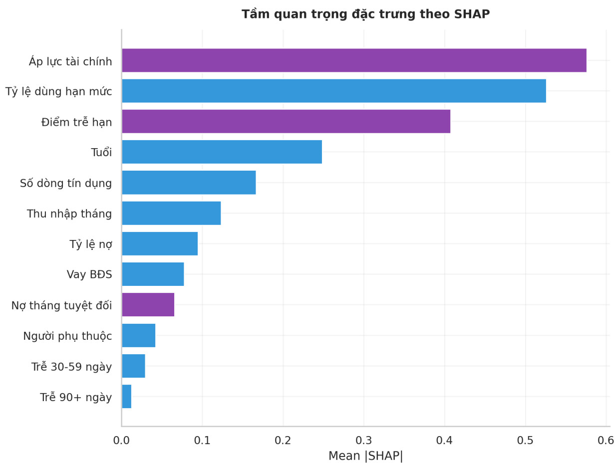
Figure 5: Tầm quan trọng đặc trưng theo SHAP
