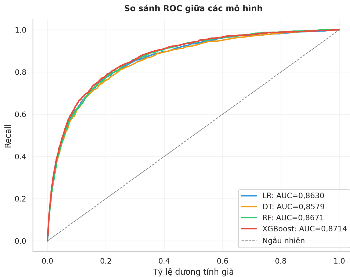
Figure 4: So sánh tổng hợp các mô hình
