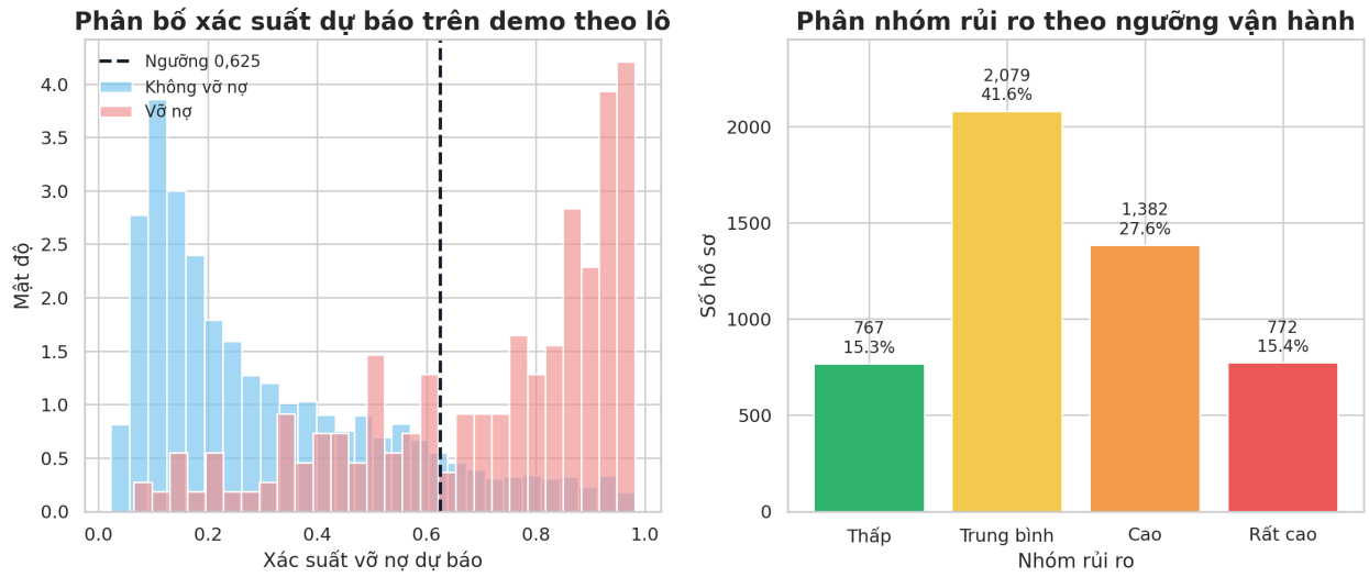
Figure 7: Phân bố xác suất và nhóm rủi ro trên demo theo lô
