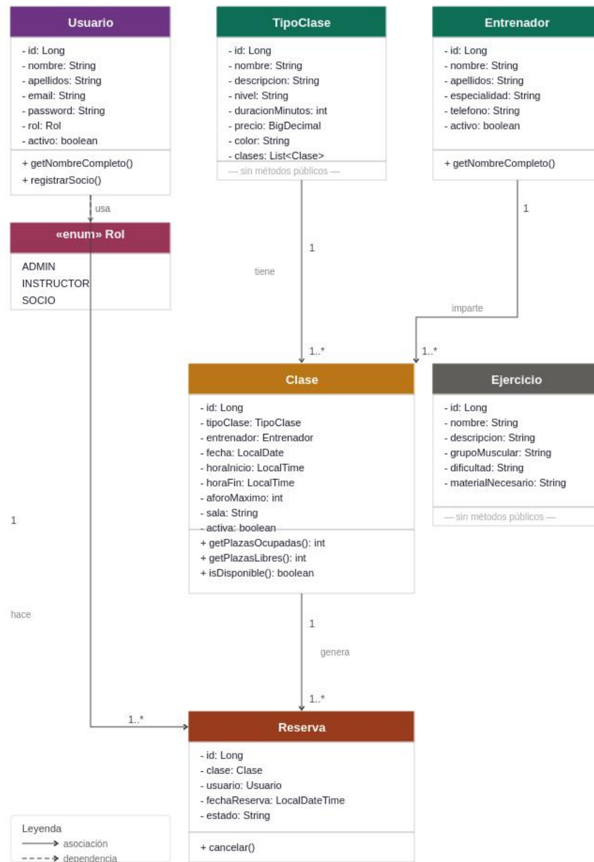
Figura UML. Diagrama de clases de PurpleForce Gym con atributos, métodos y relaciones.
