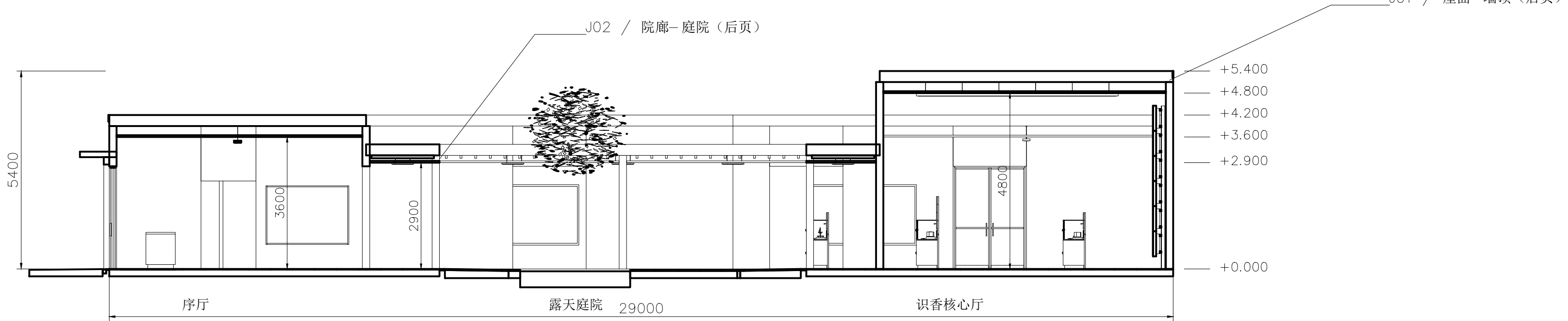
A-A x=15000 / 向西看
