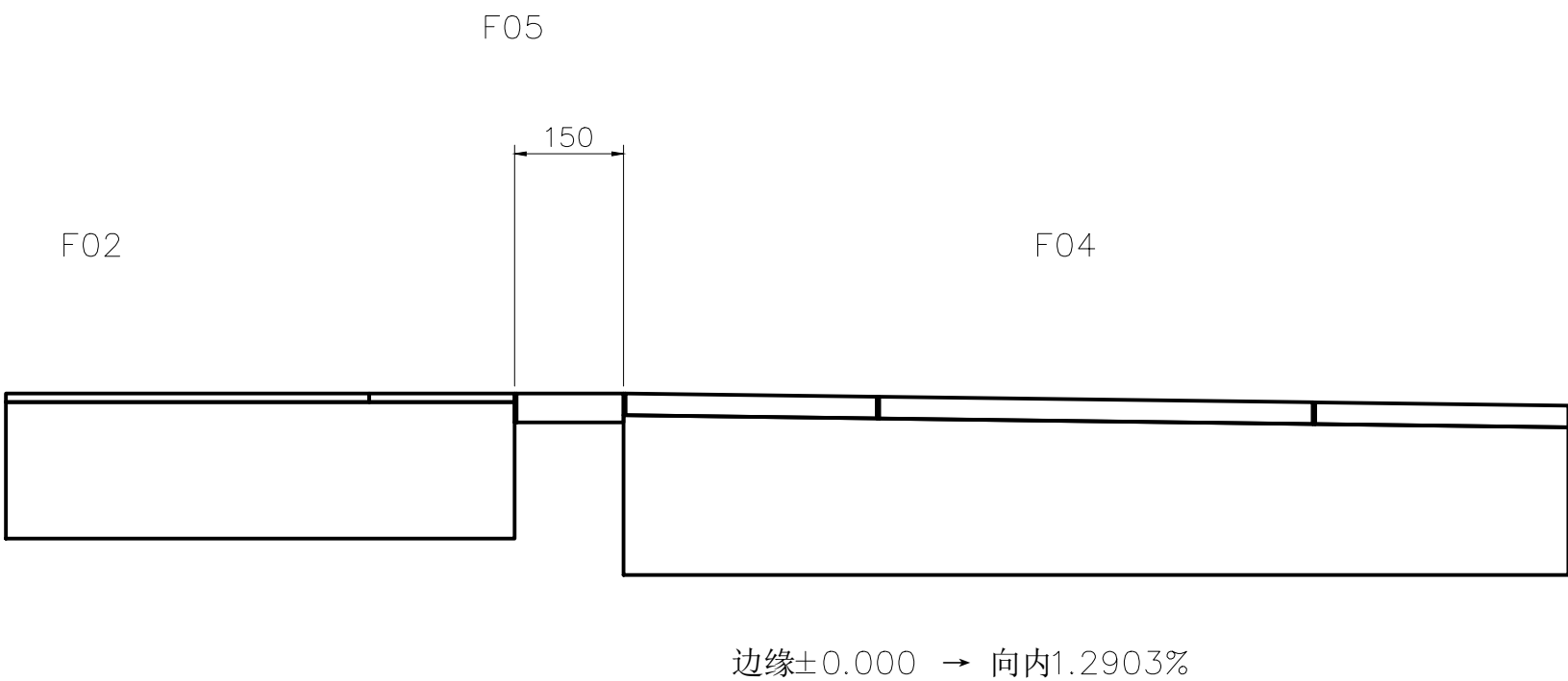
JF02 院廊 / 庭院齐平收边
