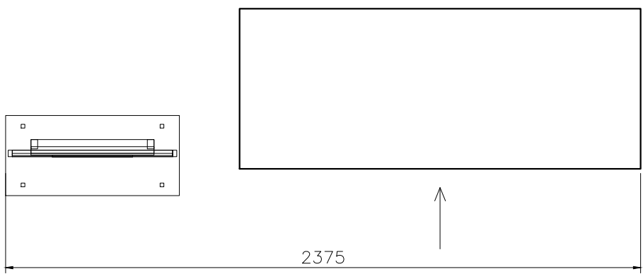
平面 / 柜身外包与图文架
