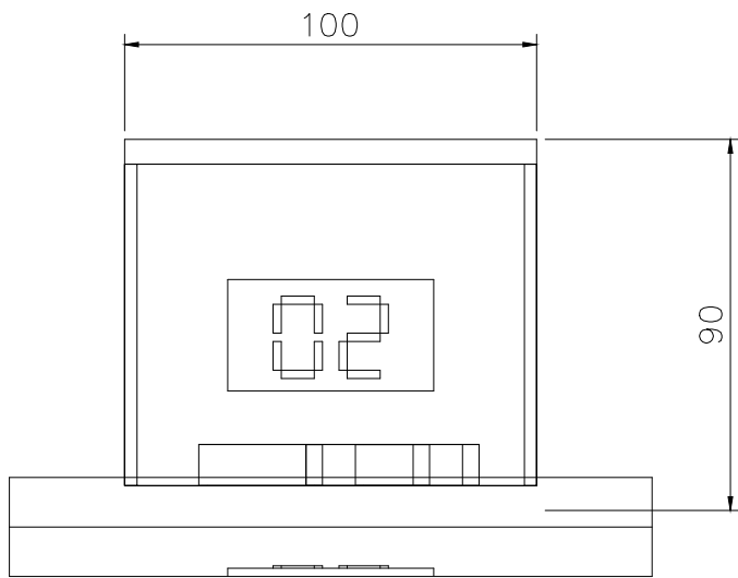
02 正视 / 90高箱体
