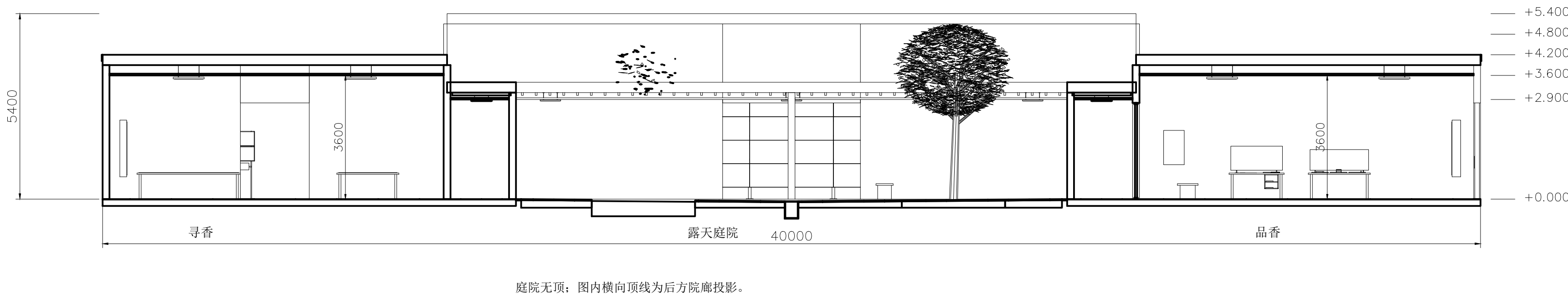
B-B y=14000 / 向北看
