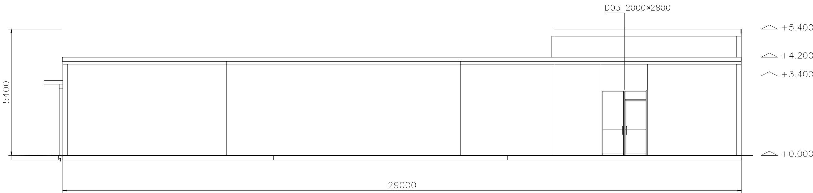
西立面 / 识香入口
