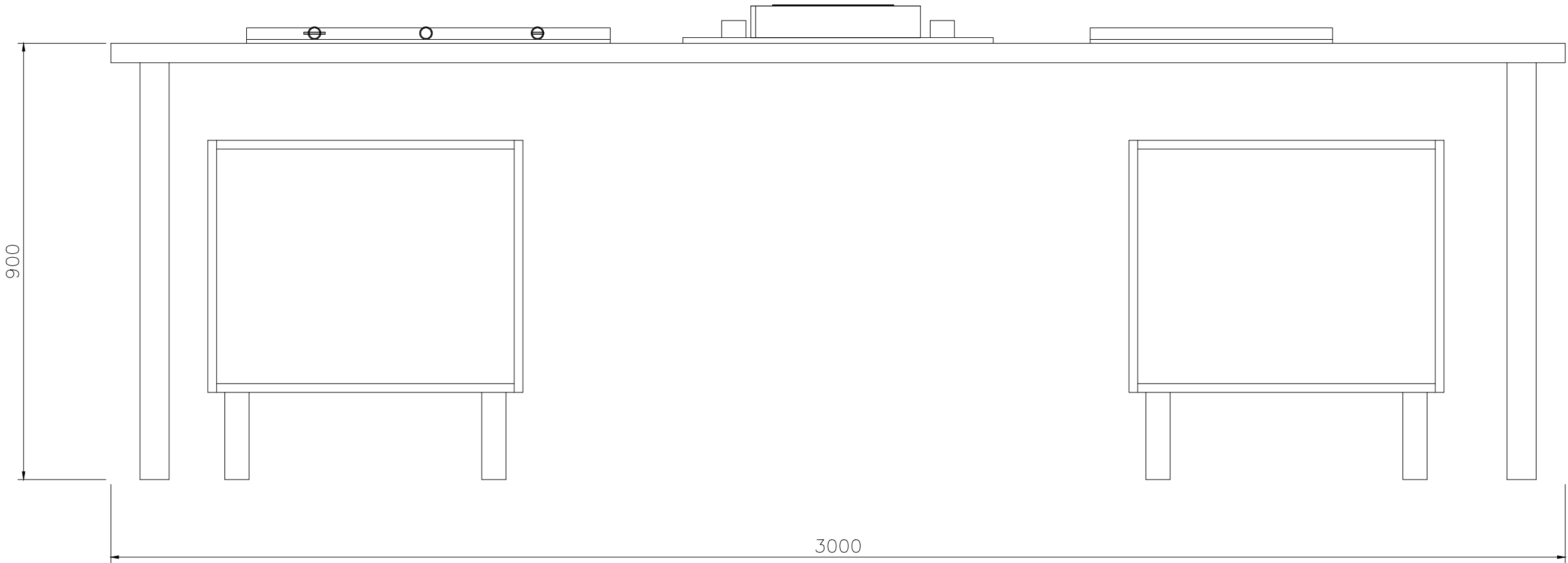
02 观众侧立面 / 储物正面向北侧
