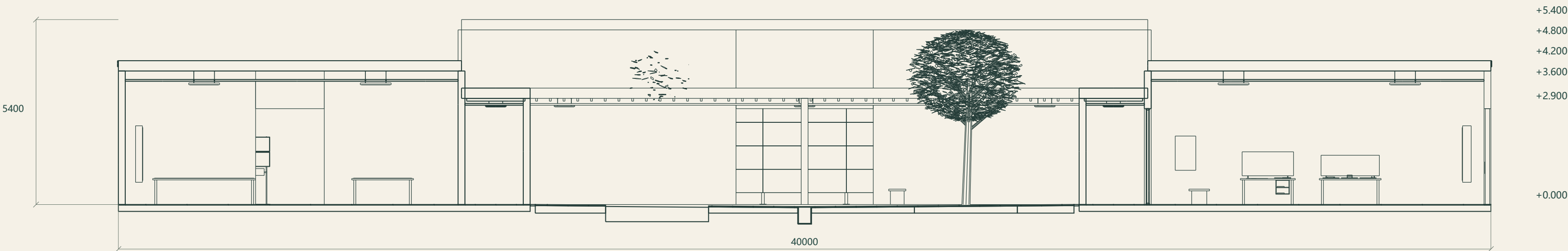
B—B 东西剖面 / 向北看 1:100
