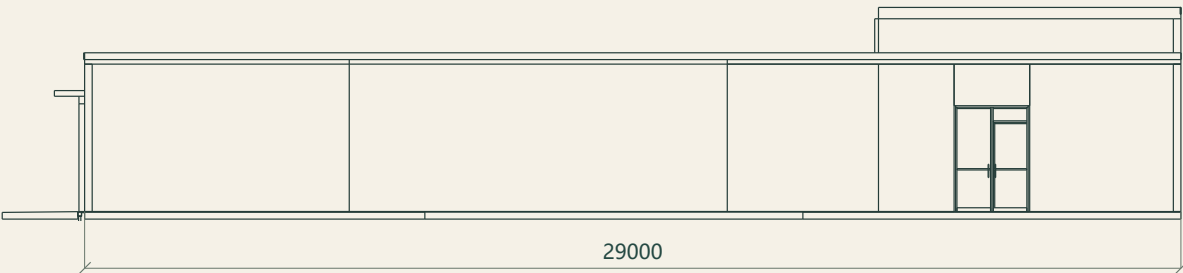
西立面 1:200
