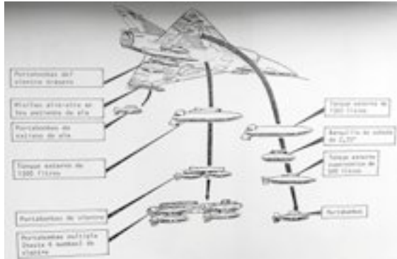
ALGUNA CONFIGURACIÓN DE LOS AVIONES DE COMBATE M5-IAI DAGGER
