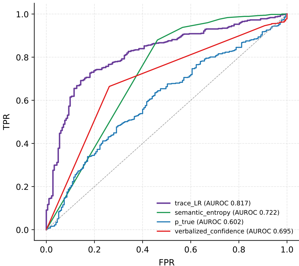
Qwen3-4B / mmlu_pro
