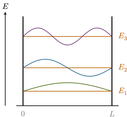
Figur 2. Uendelig dyp brønn: energinivåer E_n \propto n^2 (oransje) og tilhørende egenfunksjoner \psi_1 , \psi_2 og \psi_3 (olivengrønn, blå og plomme).
