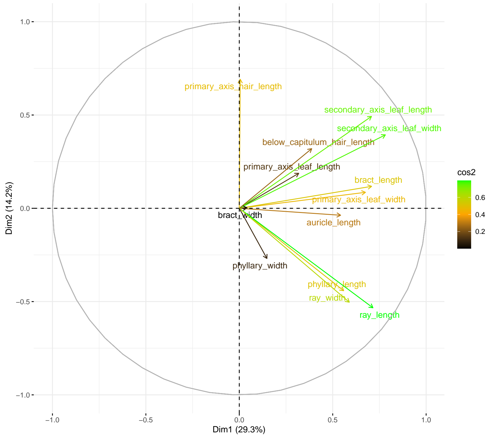
Variables – PCA
