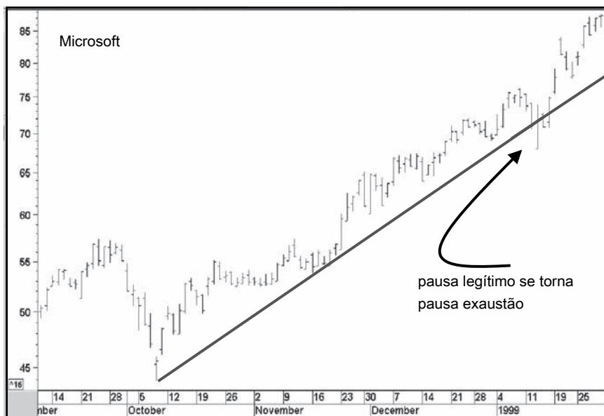
6,10 gráfico Microsoft
