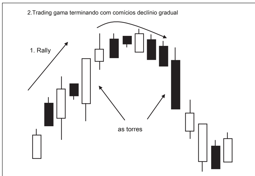
Figura 16.27 torre Top
