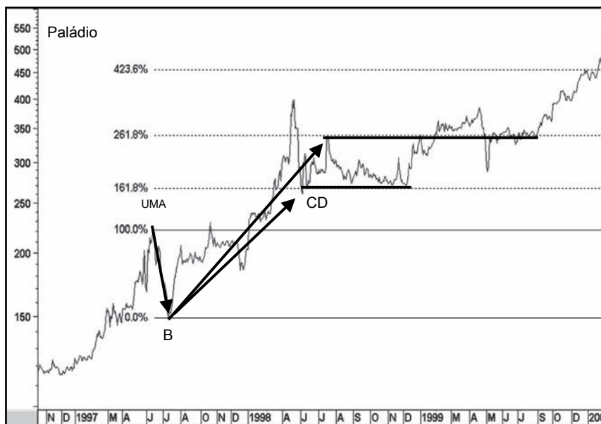
Gráfico 5.9 Paládio
