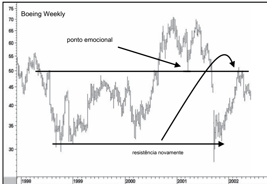
Gráfico 5.5 Boeing Weekly
