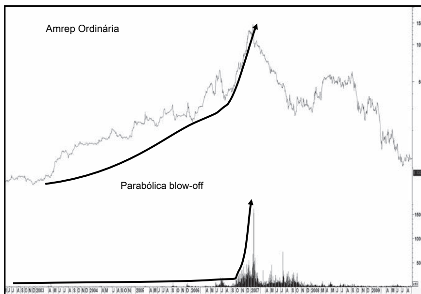
Gráfico 7.5 Amrep Ordinária 2003-2009
