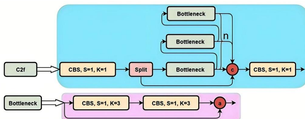
图 3.3 C2f 模块
