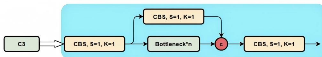
图 3.2 C3 模块
