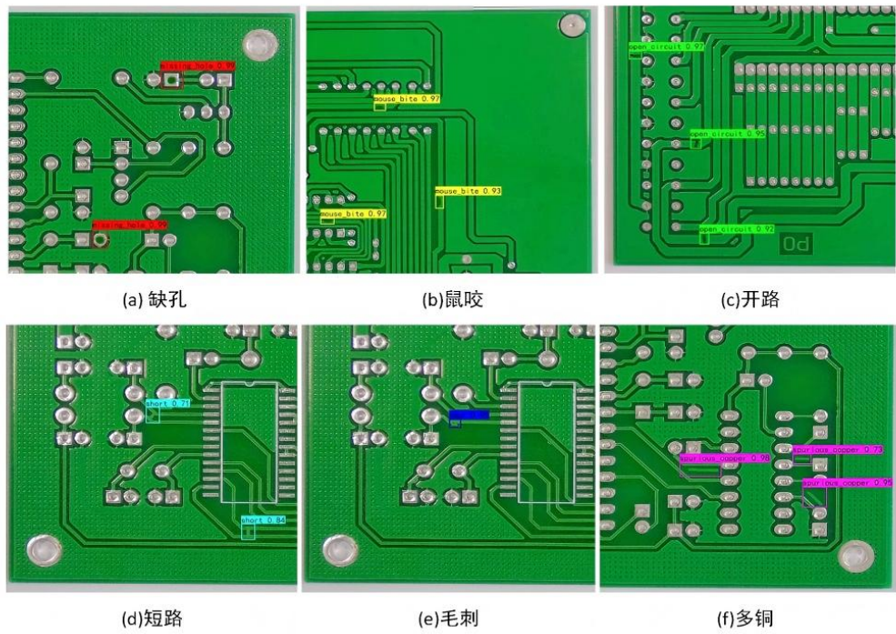
图 5.4 YOLOv8n 模型检测图
