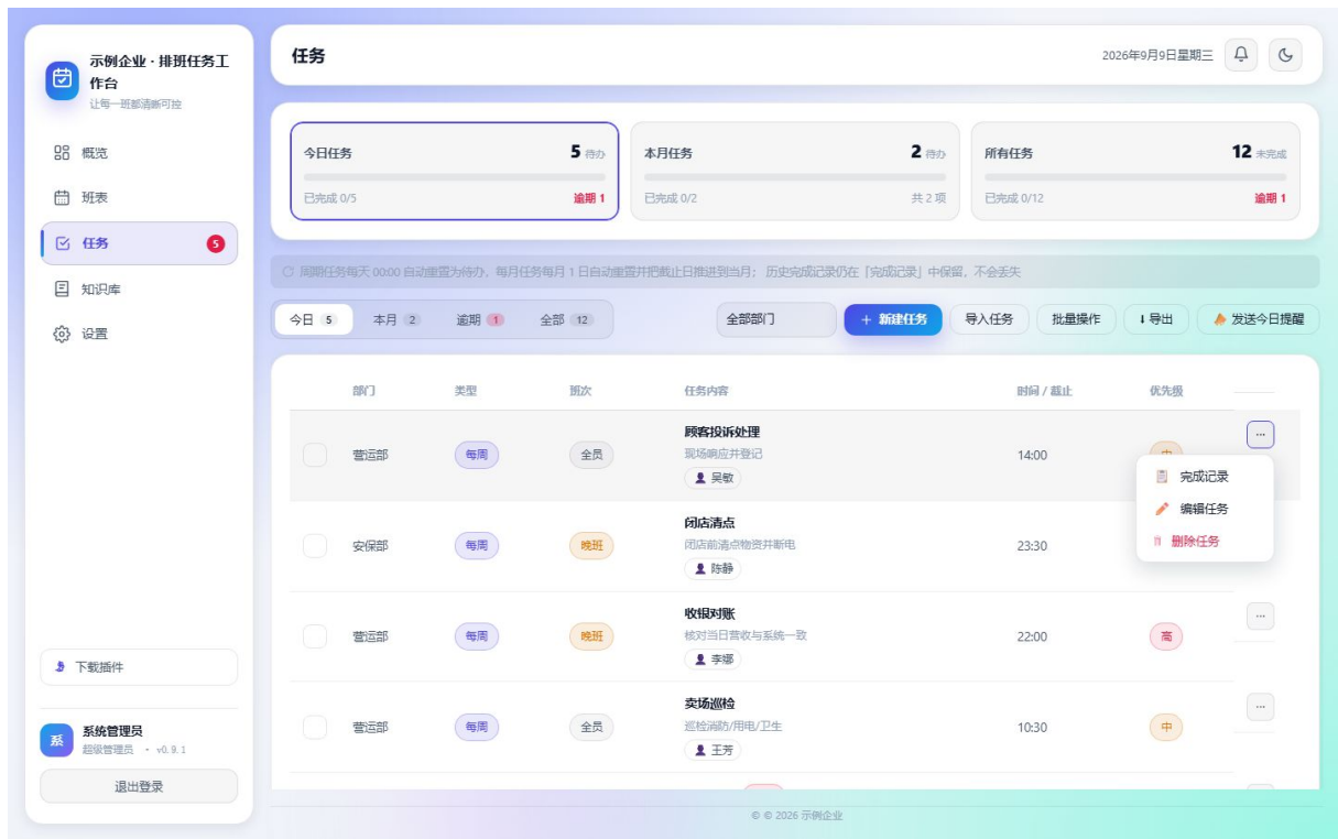
图：任务行「…」操作菜单（完成记录 / 编辑任务 / 删除任务，v0.9.1）
