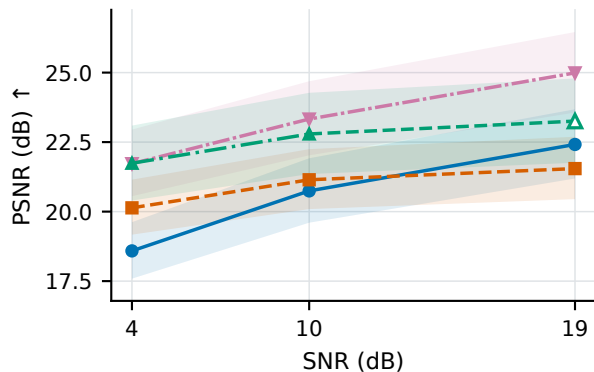
(a) PSNR
