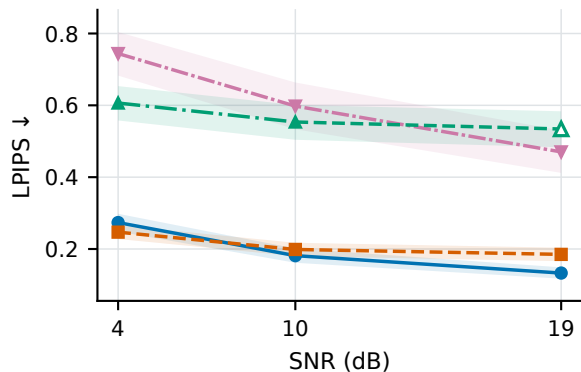
(b) LPIPS
