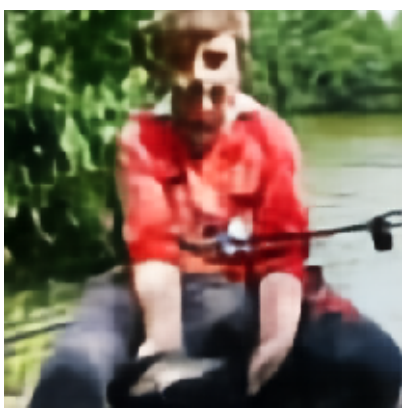
SwinJSCC
