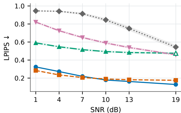
(b) LPIPS
