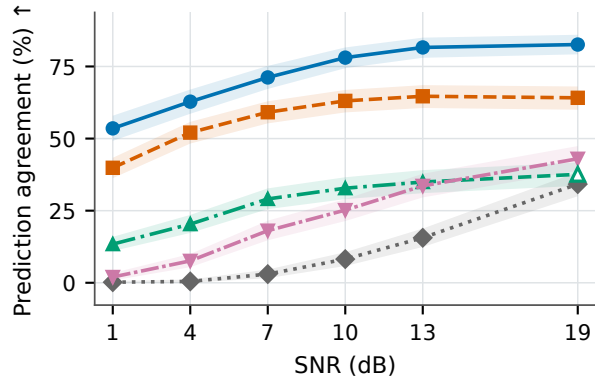
(d) ConvNeXt
