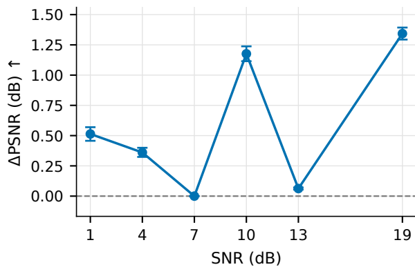
PSNR
