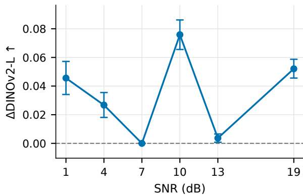
DINOv2 ViT-L/14
