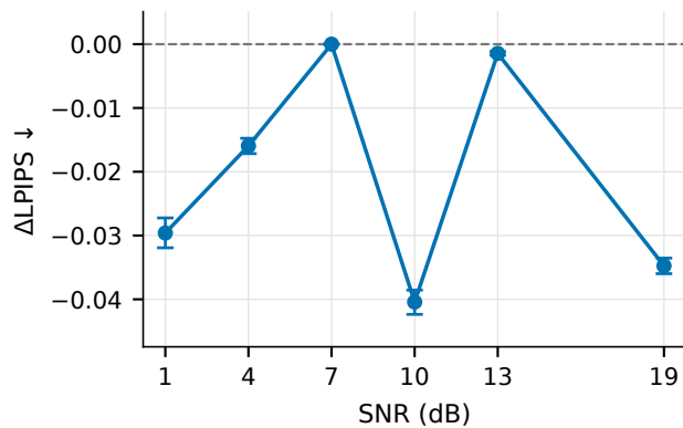
LPIPS-Alex
