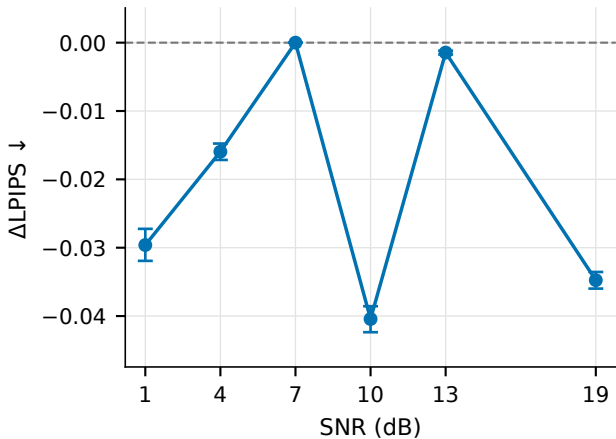
LPIPS-Alex
