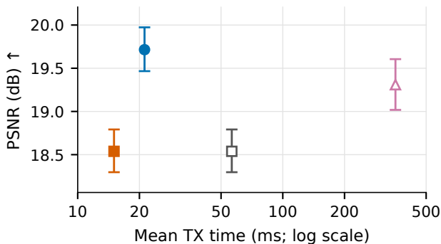
PSNR
