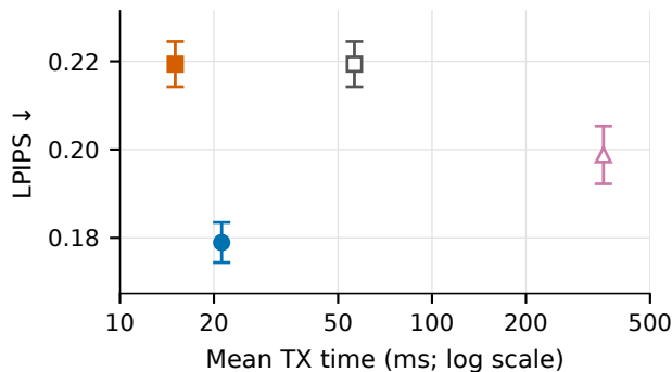
LPIPS-Alex
