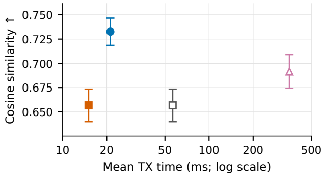
DINOv2 ViT-L/14
