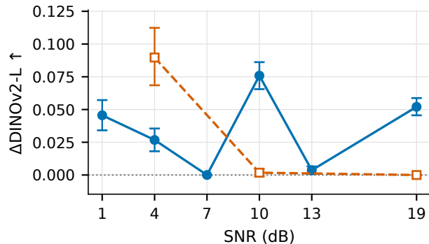
DINOv2 ViT-L/14
