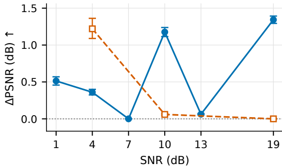
PSNR
