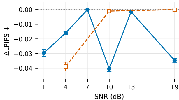
LPIPS-Alex
