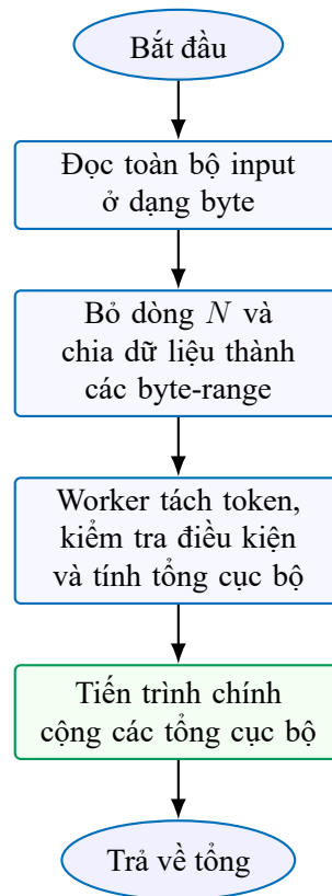
Hình 1: Luồng xử lý song song của Challenge 1
