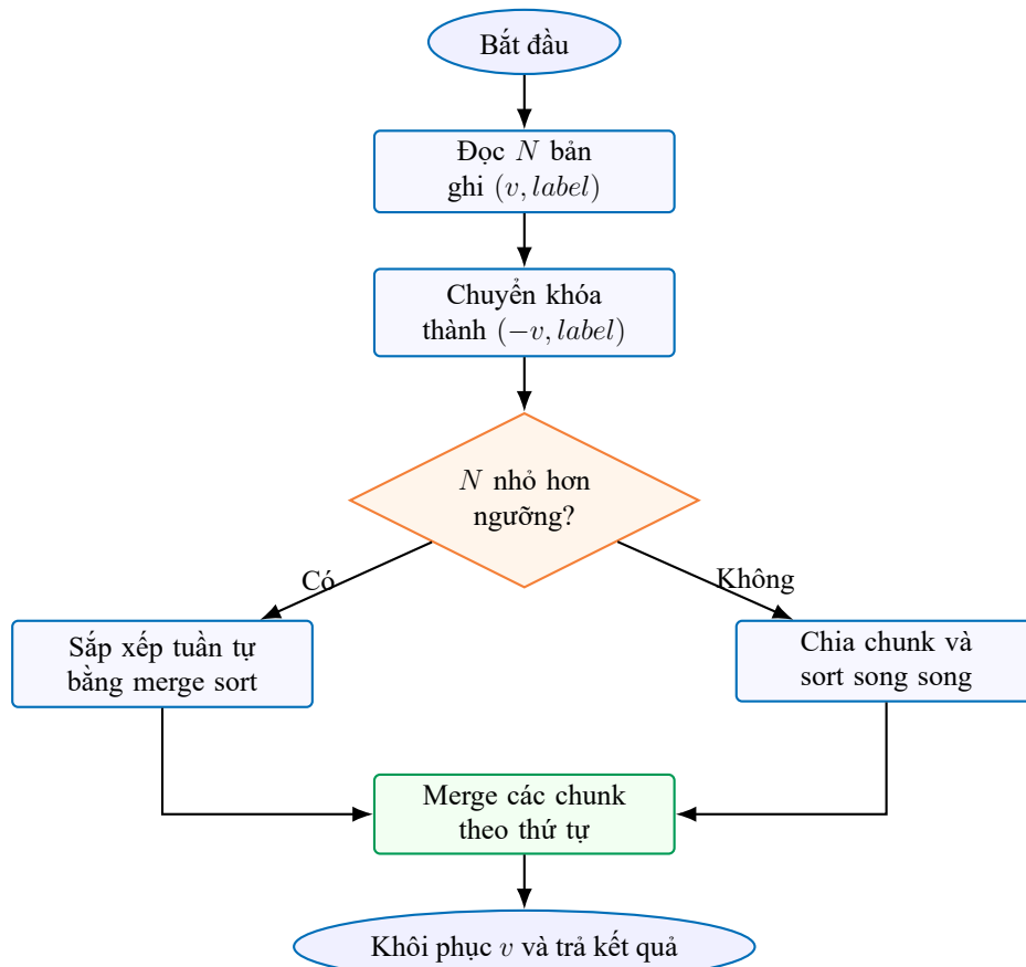
Hình 4: Luồng xử lý song song của Challenge 4
