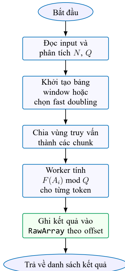
Hình 2: Luồng xử lý song song của Challenge 2
