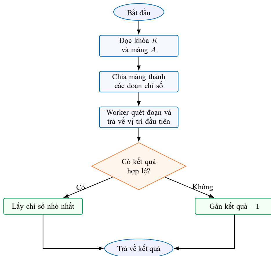
Hình 5: Luồng xử lý đề xuất cho Challenge 5
