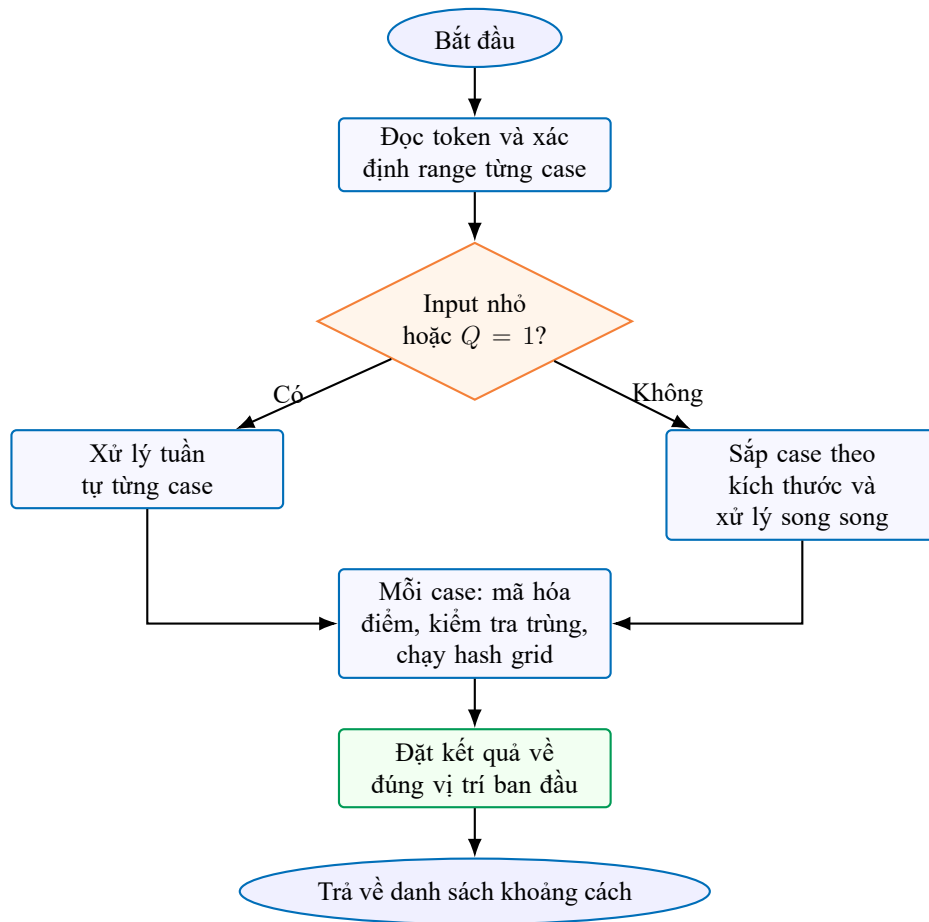
Hình 6: Luồng xử lý song song của Challenge 6
