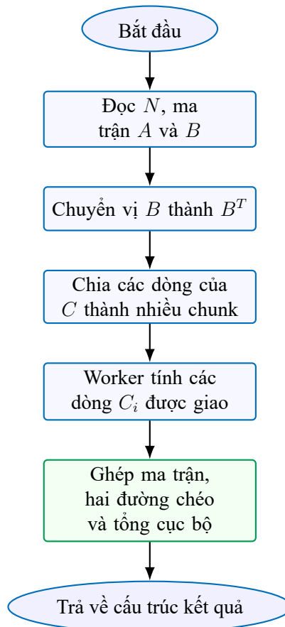
Hình 3: Luồng xử lý song song của Challenge 3
