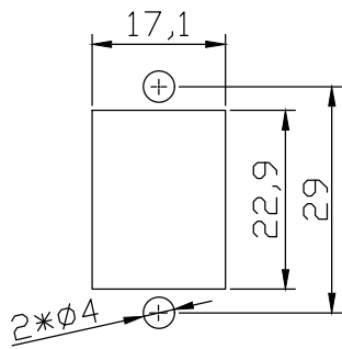
开孔尺寸 (单位: mm)
