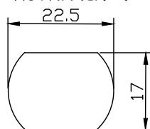
〈止转安装开孔方式〉
