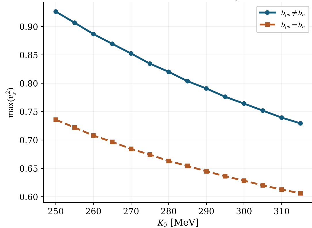
Peak beta-equilibrium v_s^2
