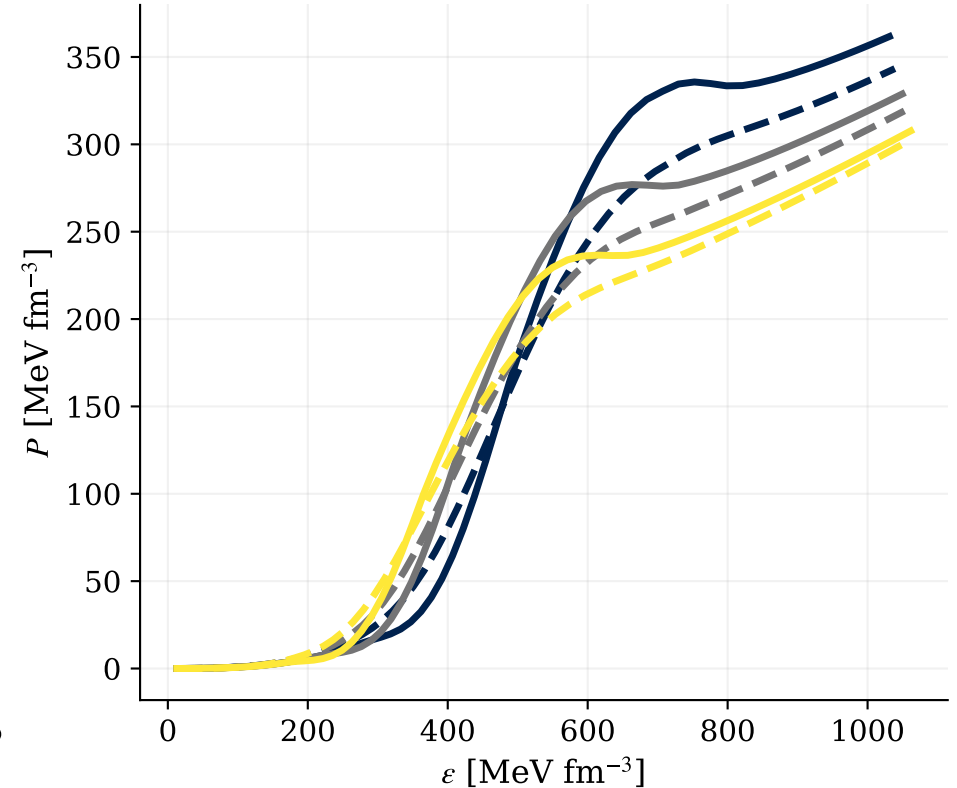
Beta-equilibrium EOS
