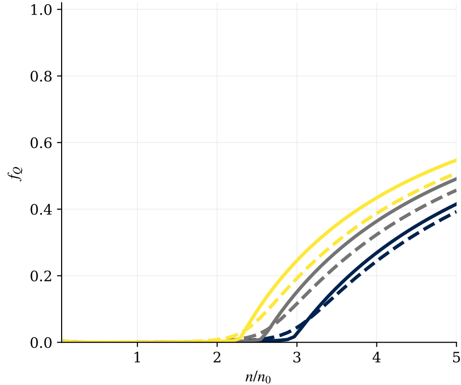
Beta-equilibrium EOS
