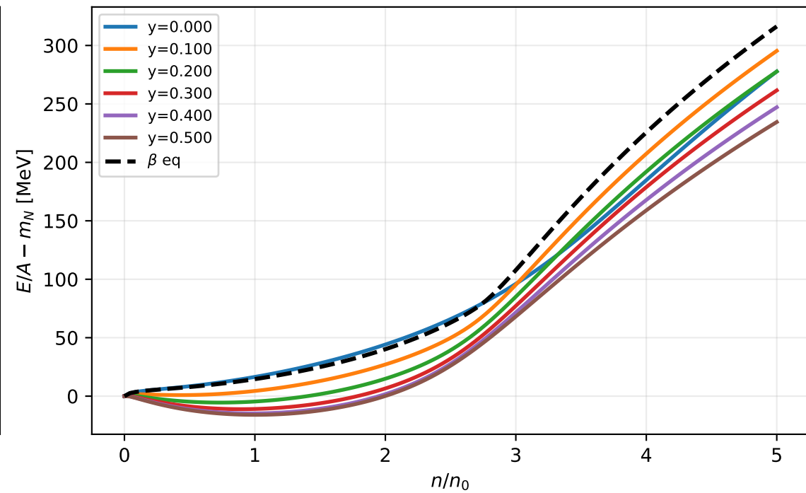
E/A - m_N
