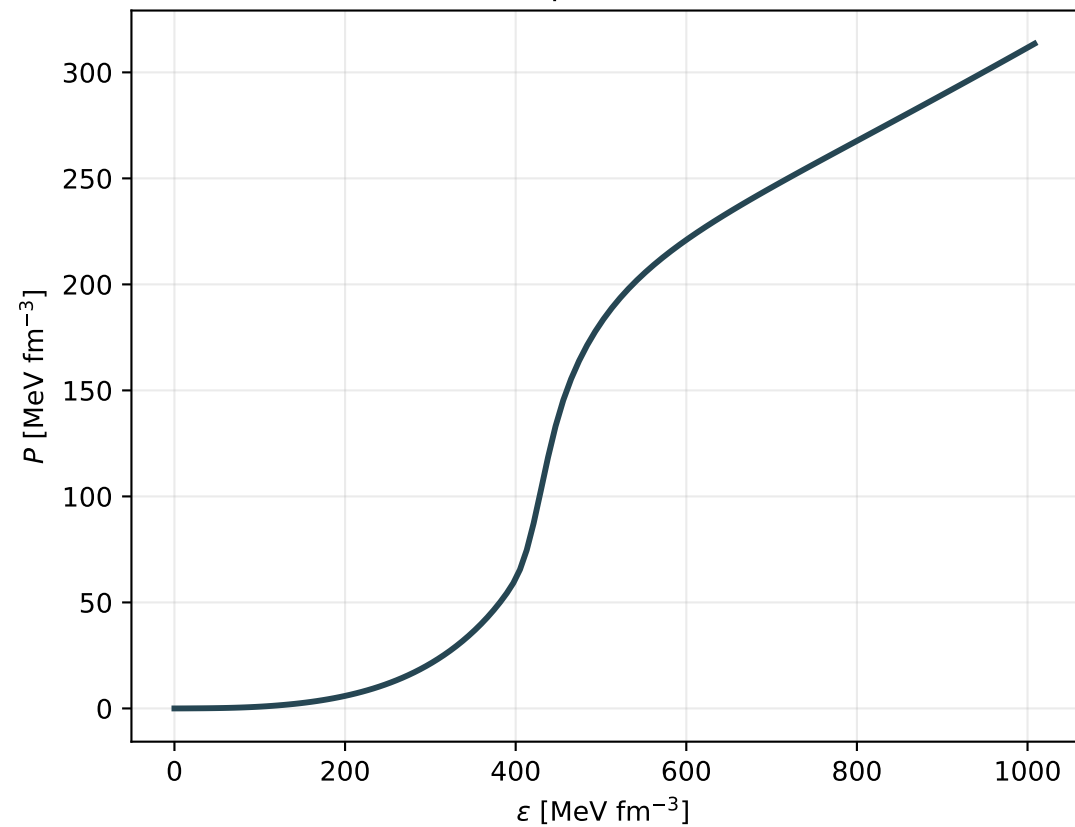
Beta-Equilibrium EOS
