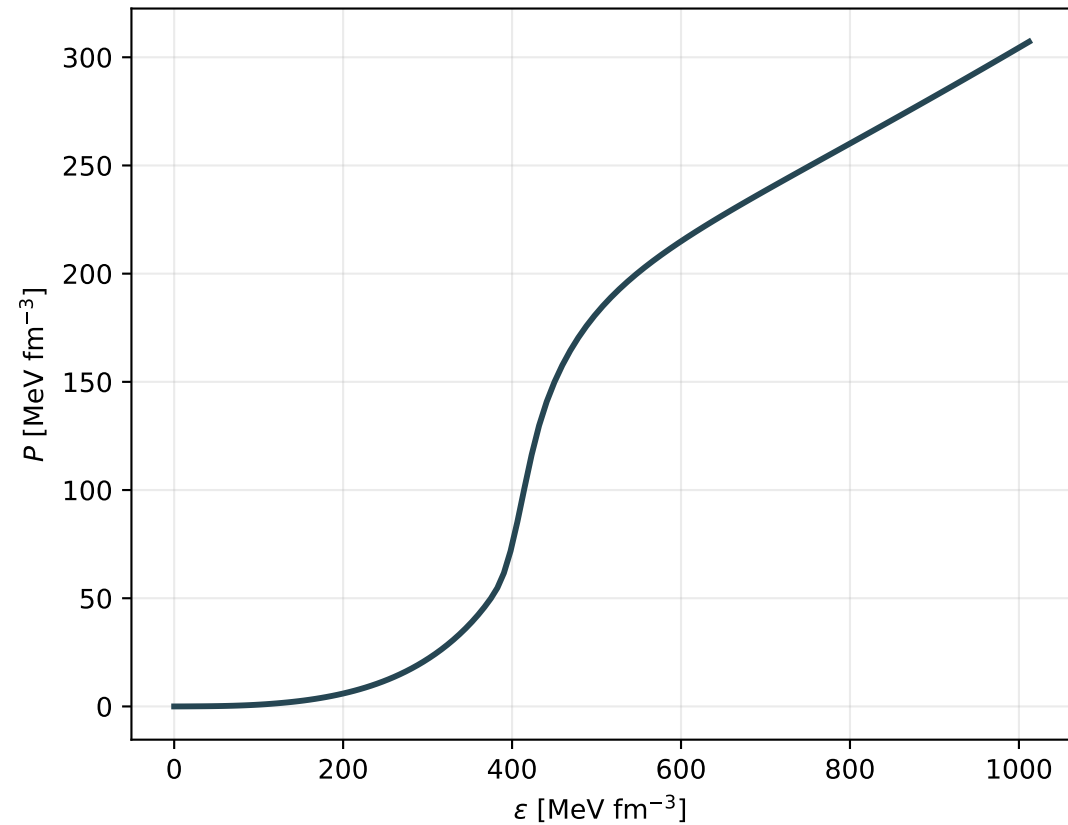
Beta-Equilibrium EOS
