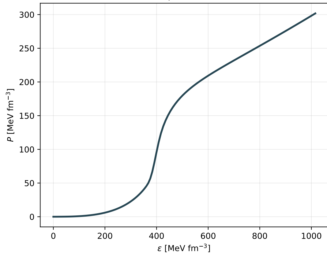
Beta-Equilibrium EOS
